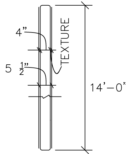
6 PANEL CROSS SECTION N.T.S
